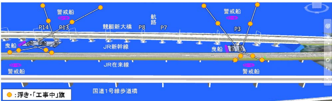
P13~P14: 台船を橋脚間に配置
