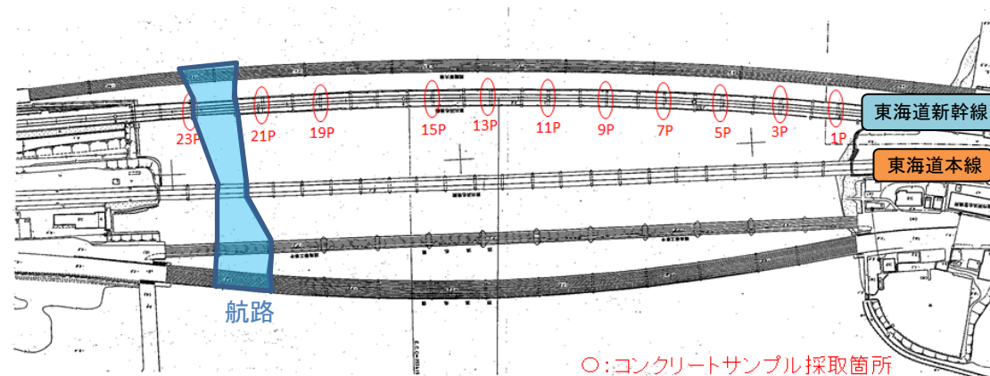
【詳細図】
